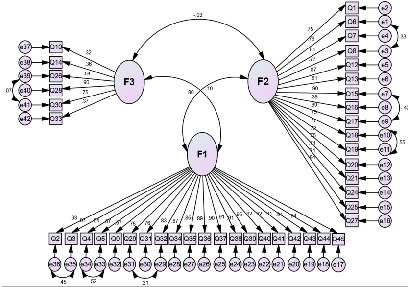
شكل (٢) التقديرات المعيارية التحليل العاملي التوكيدي لمقياس المساندة الاجتماعية باستخدام AMOS (V_21)
