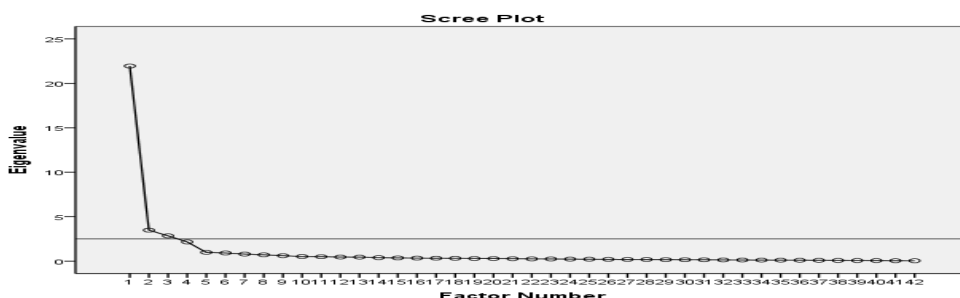
شكل (١) منحنى تشبعات المكونات العاملية للمقياس (scree plot)
